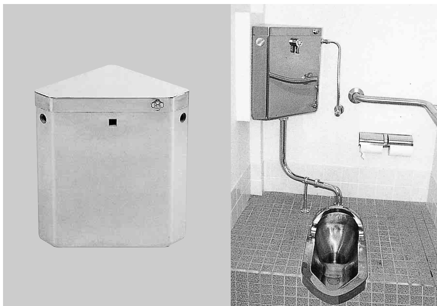
コーナー型ロータンクM-1001型と完成例（便器は和式大便器上給水型）
