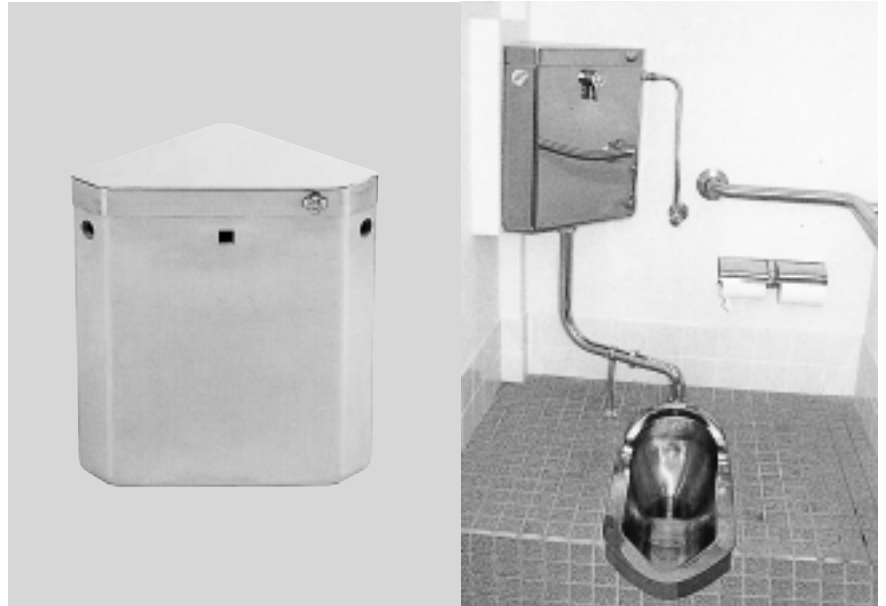
コーナー型ロータンクM-1001型と完成例（便器は和式大便器上給水型）
