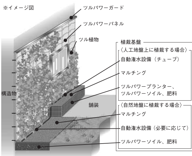
東京都壁面緑化モデル 省メンテナンス型の壁面緑化システムとして採用 (H=16m、東京都千代田区)
