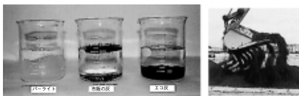
エコ炭攪拌状況 (飛散しにくい)
